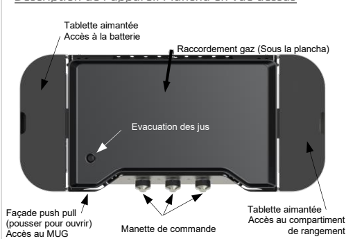
Description de l'appareil Plancha en vue dessus
