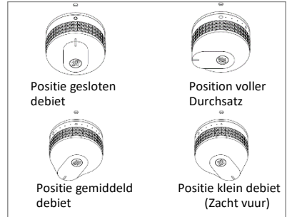
Figuur 2: Regeling van de bedieningshendel
